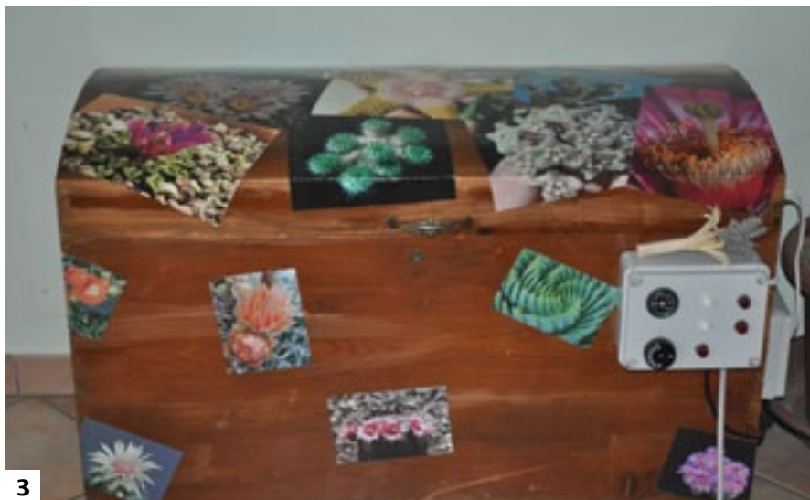
1 · Il primo germinatoio. 2 · rivestimento in polistirolo e cavo scaldante sotto l'argilla espansa. 3 · Scatola del termostato con manopola di regolazione della temperatura. 4 · Il secondo germinatoio. 5 · Interno del secondo germinatoio con carta argentata, termometro, cavo scaldante.
